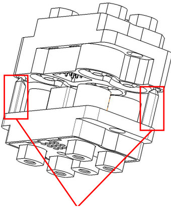
Guide Pillars
