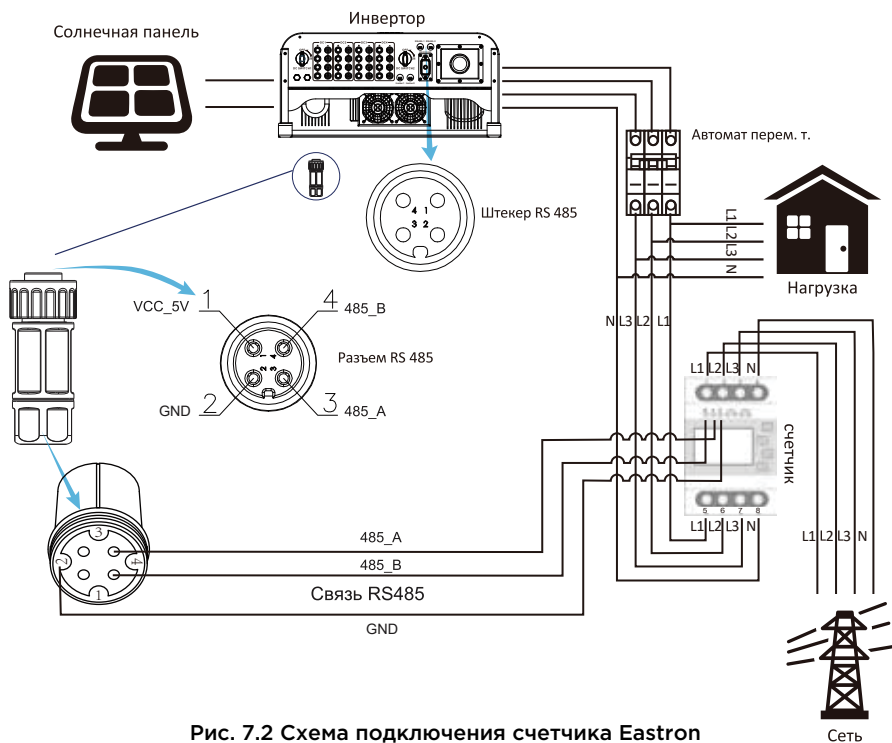
Рис. 7.2 Схема подключения счетчика Eastron
