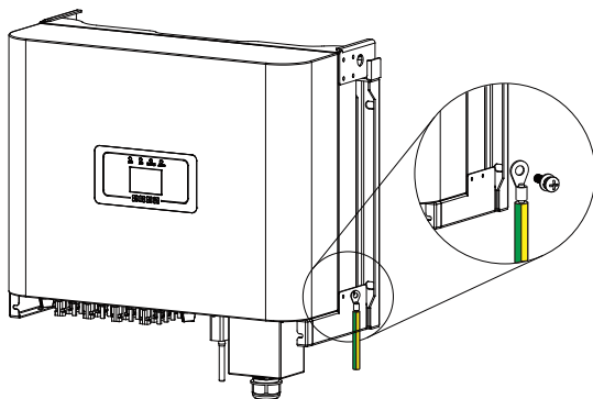
Рис. 5.12 Подключение кабеля заземления
