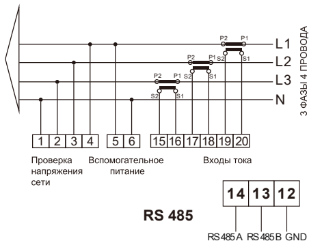
Рис. 7.12 Счетчик Eastron
