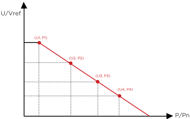
Рис. 8.28 Кривая регулирования активной мощности в режиме PU
