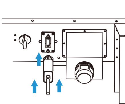
Рис. 5.14 Схема установки регистратора данных
