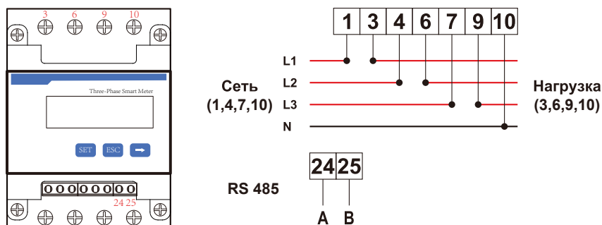
Рис. 7.5 Счетчик CHNT
