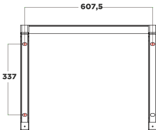
Рис. 4.3 Зазор при установке
