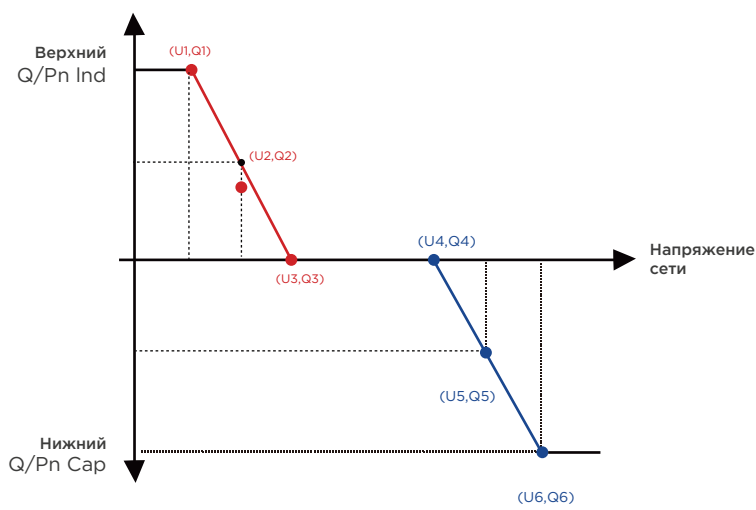
Рис. 8.26 Кривая регулирования реактивной мощности в режиме Q (U)
