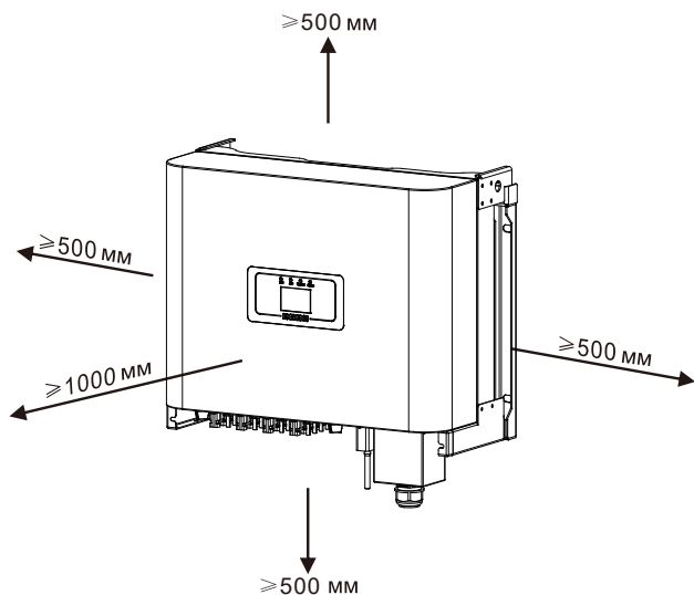
Рис. 4.3 Зазор при установке
