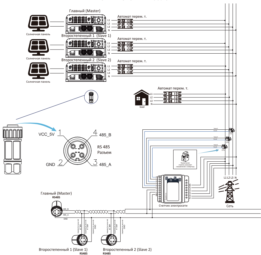
Рис. 7.13 Схема подключения (три фазы)
