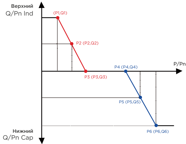
Рис. 8.27 Кривая регулирования реактивной мощности в режиме Q (P)
