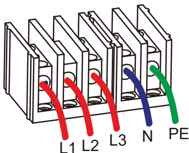
Рис. 5.9 Кабель перем. тока, подключенный входным клеммам
