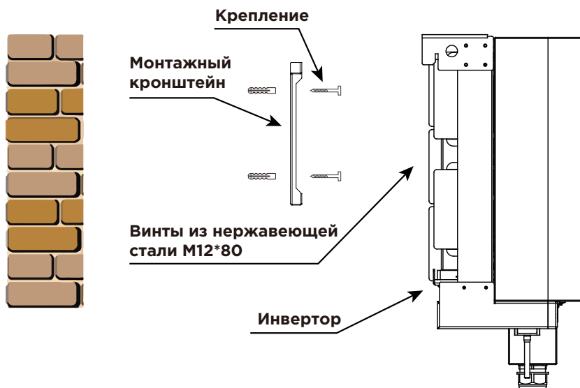
Рис. 4.5 Установка инвертора
