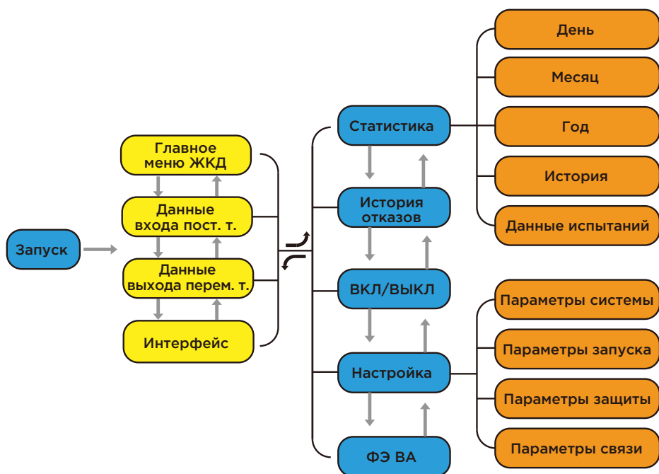
Схема меню дисплея
