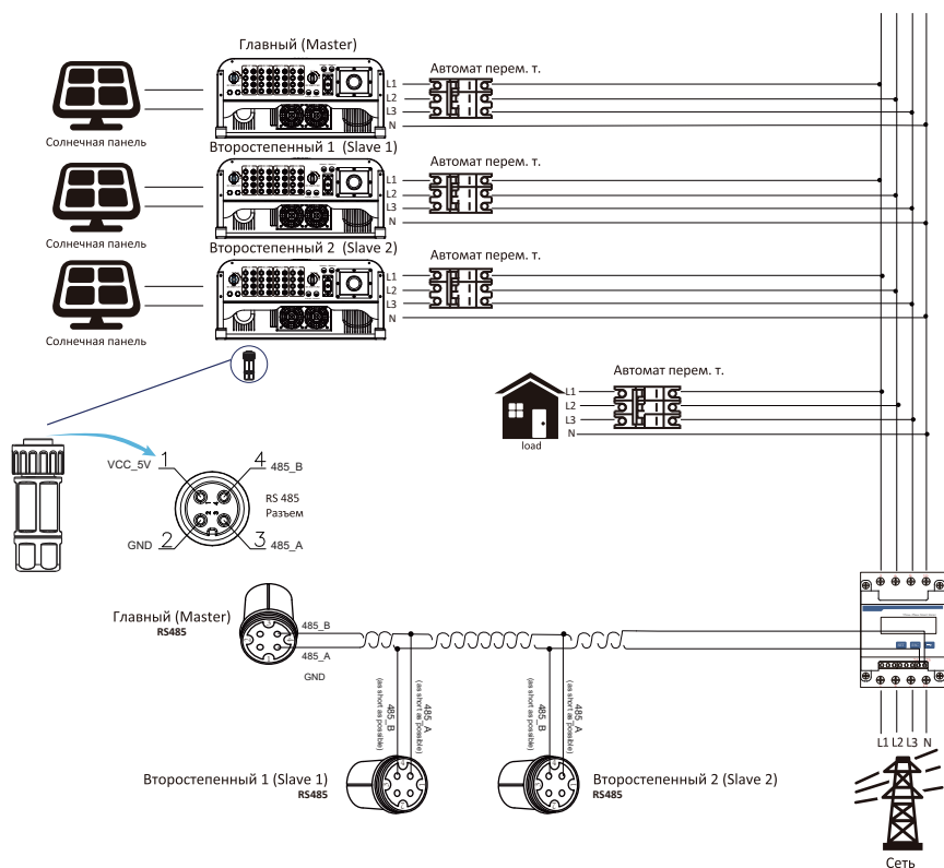
Рис. 7.15 Схема подключения CHNT (проходная схема)
