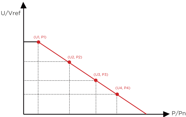
Рис. 8.28 Кривая регулирования активной мощности в режиме PU
