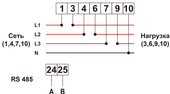
Рис. 7.5 Счетчик CHNT
