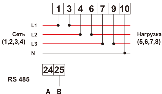
Рис. 7.14 Счетчик CHNT
