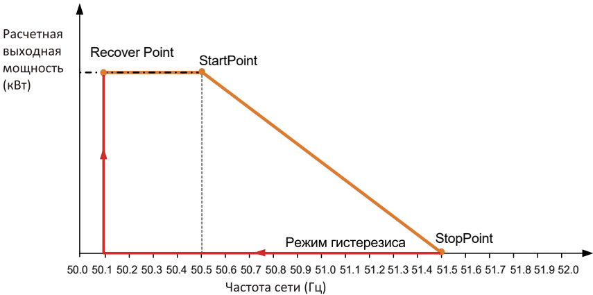
Режим частоты / мощности для условия превышения частоты
