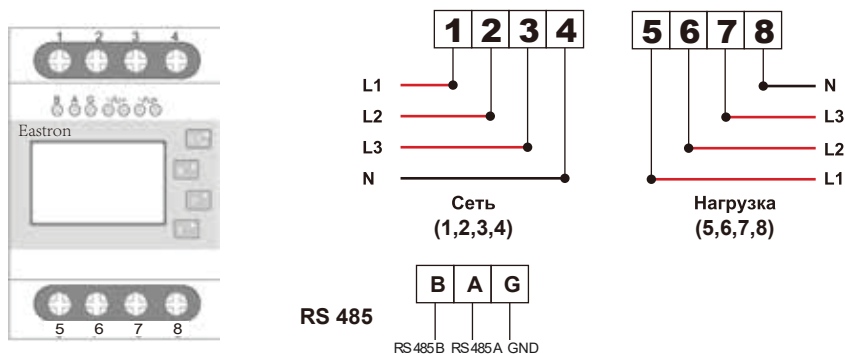
Рис. 7.10 Счетчик Eastron
