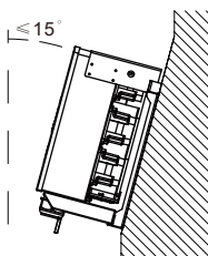
Рис. 4.2 Угол установки
